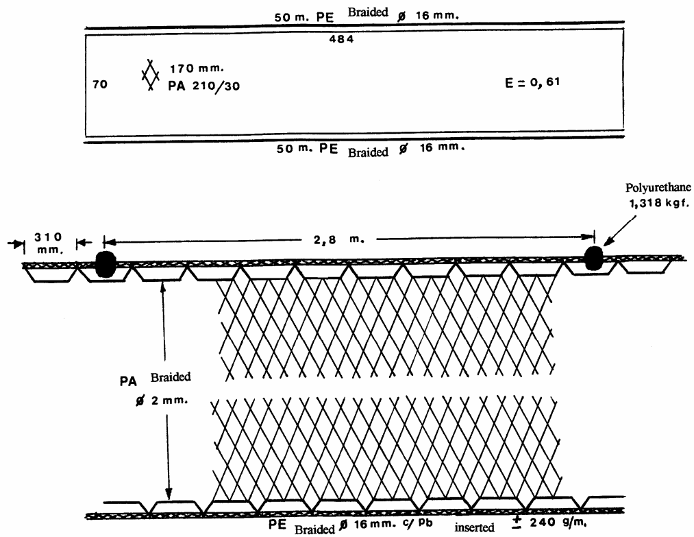
FIGURA 25 – Modelo de rede de emalhe de superfície utilizada para capturar tubarões-martelo. Frota sediada em Itajaí e Navegantes (SC). Ano 1995. Desenho de autoria de Manoel da Rocha Gamba.
