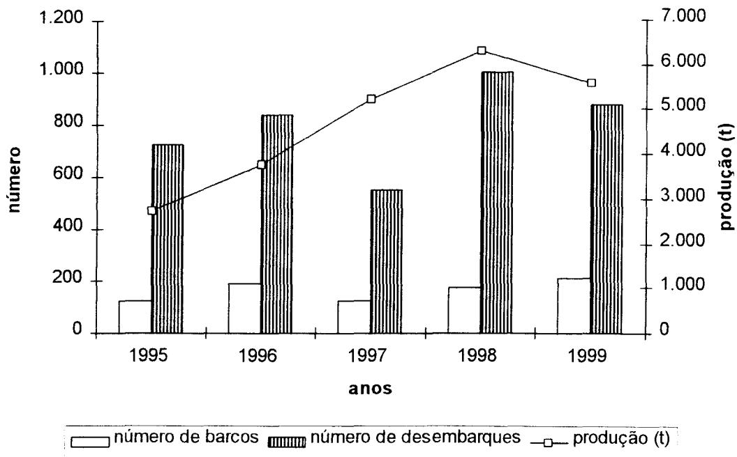
Figura 3 – Pesca de Arrasto de Camarão
