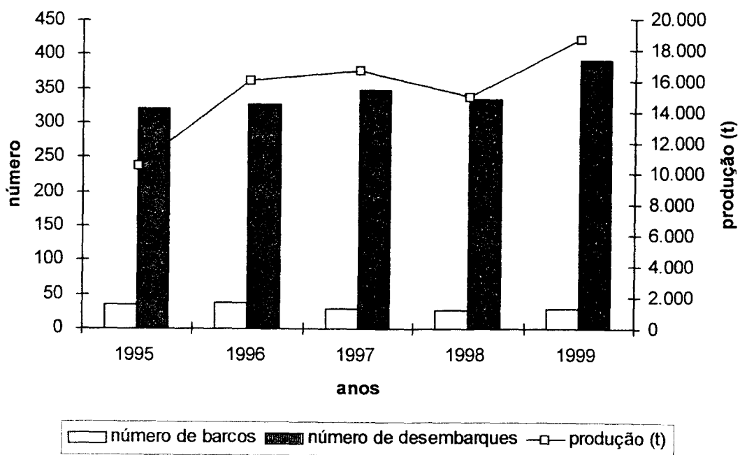
Figura 6 - Pesca de Vara e Isca-viva
